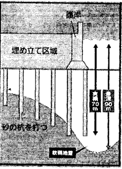
大浦湾の軟弱地盤を改良できない埋め立て工法 (出典:埋めるな!連のリーフレット)
